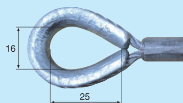
アイ加工済みワイヤー（標準装備）の寸法
